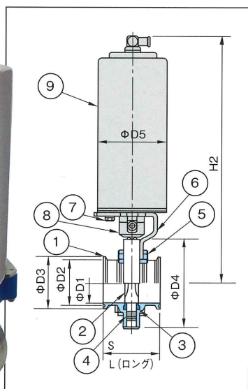
■ ZK668 (自動式) 寸法表
